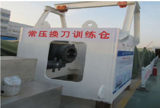
常压换刀训练仓
