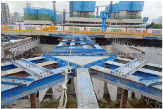
新型钢支撑
