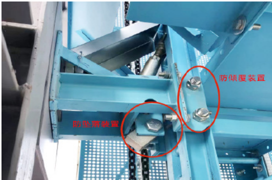
防坠落、防倾覆装置
