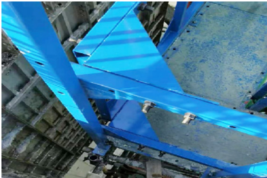
转角处水平桁架连接
