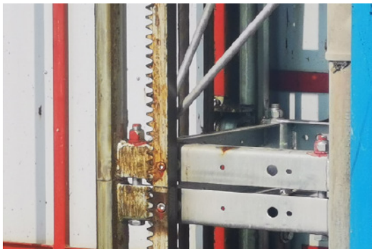
导轨架防松螺栓及油漆标记
