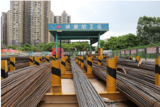
钢筋加工区
