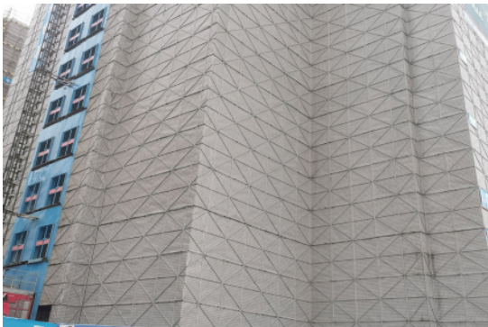
脚手架采用钢防护网外立面
