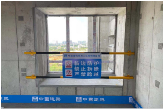
窗口临边防护
